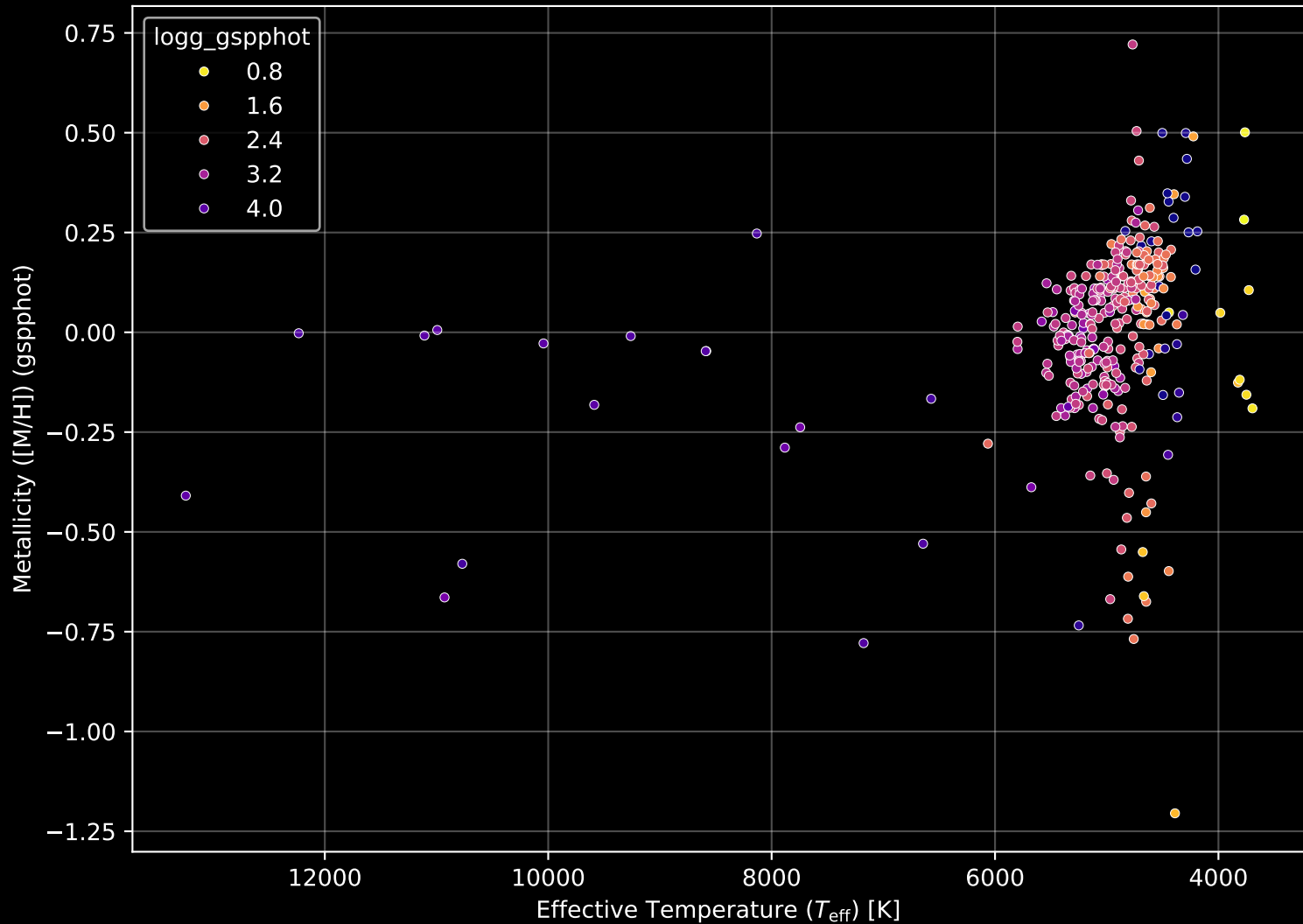
APOGEE DR17 Field: [140+12] Stellar Population Parameters (n= 352)
